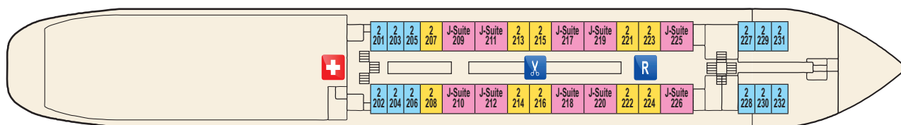
Hauptdeck / Deck 2
